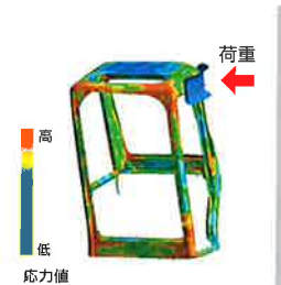
ROPS応力解析図
