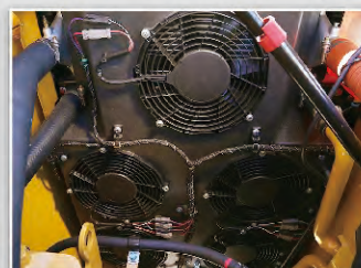
逆転機能付電動クーリングファン
